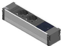
Varenr: LPBOXE Kabelboks 2 x 230 V, 1 x USB C, 30 W
