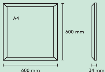
Väggpanel A4 / Wall panel A4 / Wandpaneel A4
