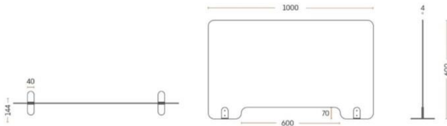
SMITTEAFSKÆRMNING MED UDSKÆRING 5000-0013-9005
