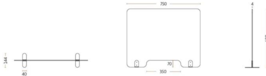
SMITTEAFSKÆRMNING MED UDSKÆRING 5000-0013-9005
